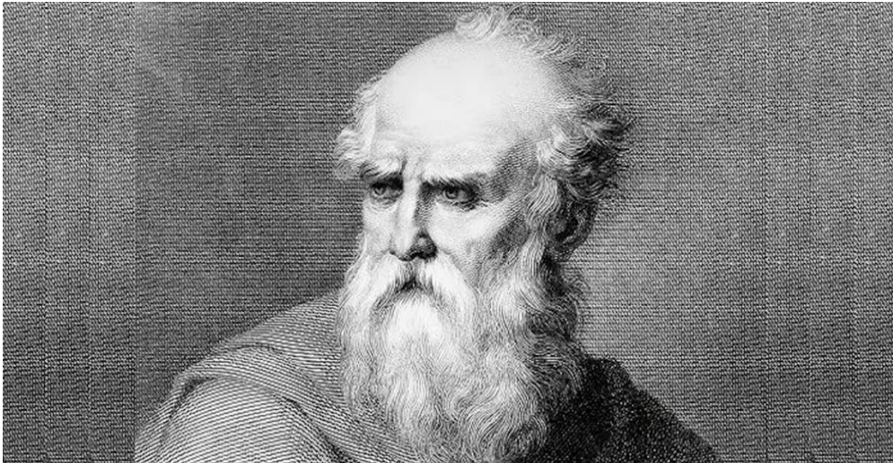
Afbeelding Vitruvius MooiNL
